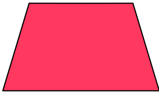
trapezium
